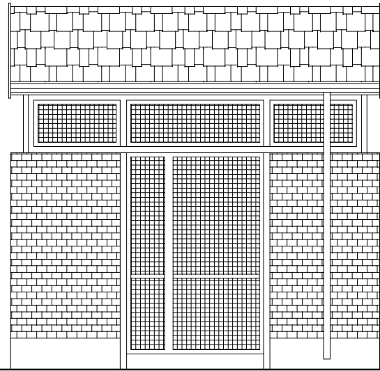
ELEWACJA PRZEDNIA
