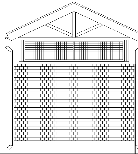
ELEWACJA BOCZNA
